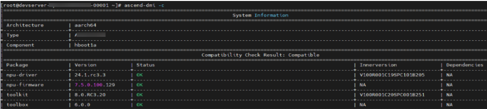
图 8-7 软硬件版本兼容性测试示例
